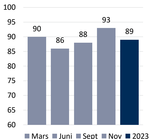
Figur 7 HME-mätningar 2023
