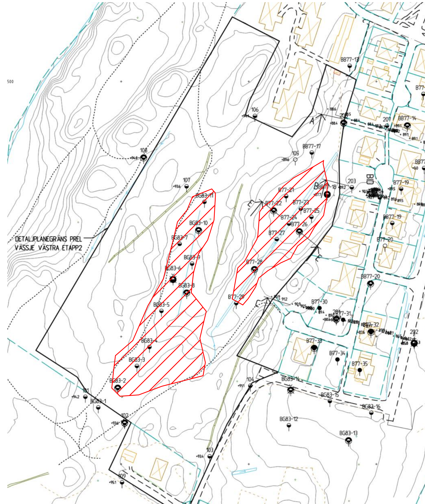
De huvudsakliga områdena med dy, gytta eller torv i de ytliga jordlagren.
